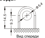
Вид спереди
