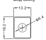
Вид сверху
